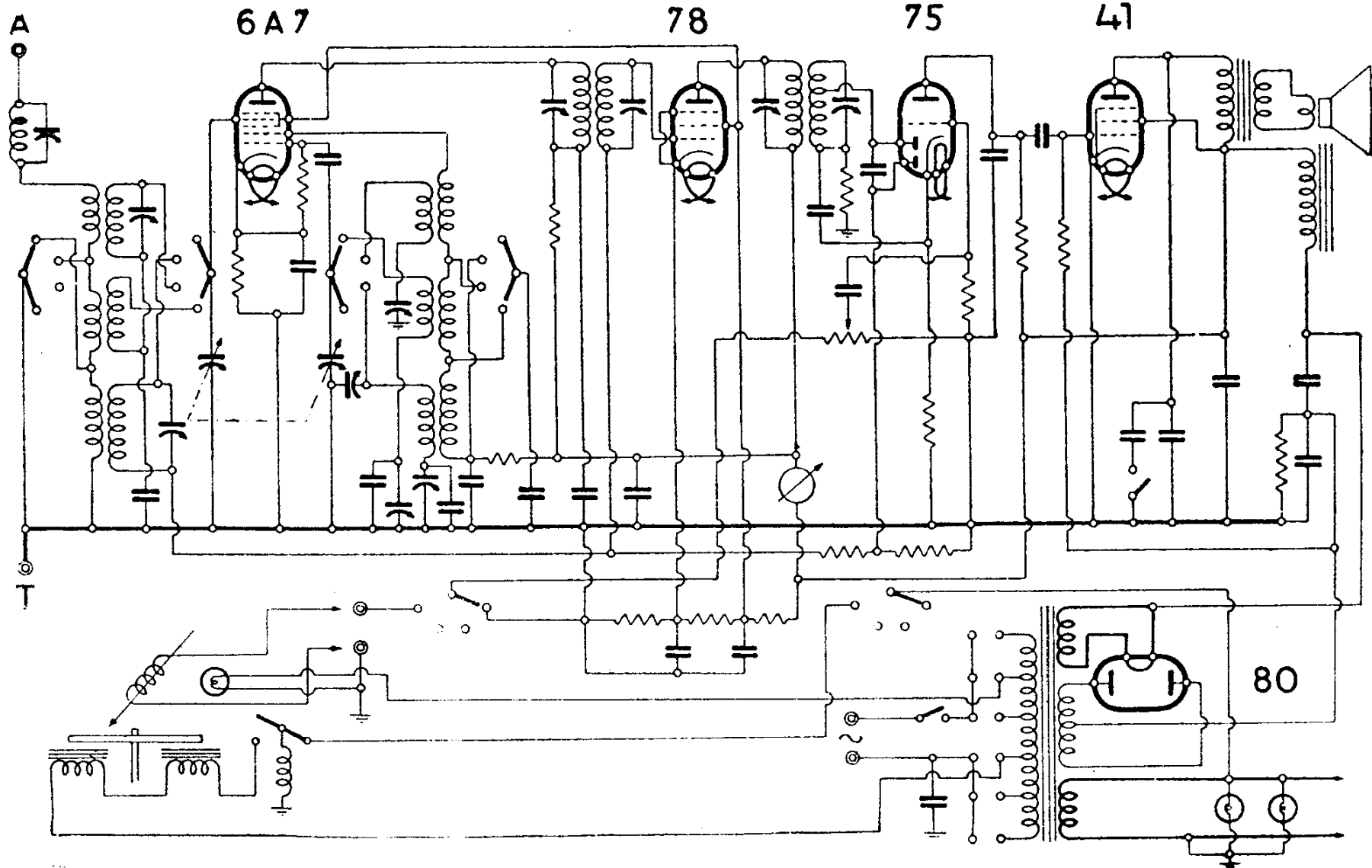
RADIOMARELLI - MOD. « FALTUSA »
